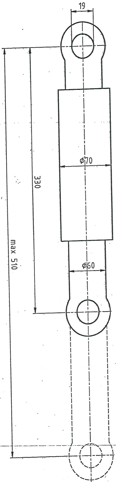
Skica 1 - Amortizer za podvozak M-832
