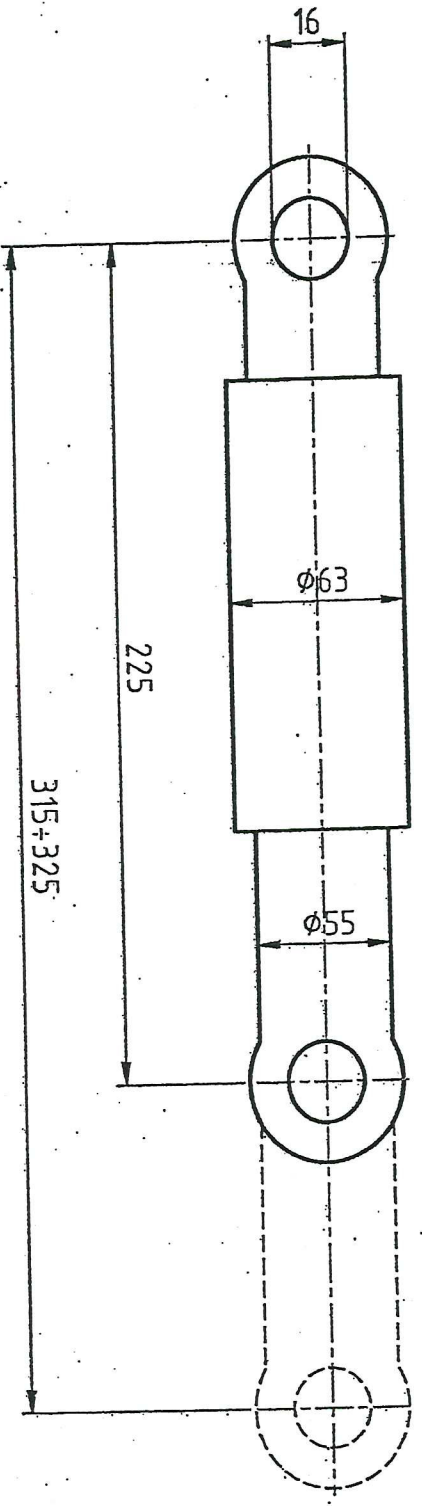
Skica 2 - Amortizer za podvozak A-6000
