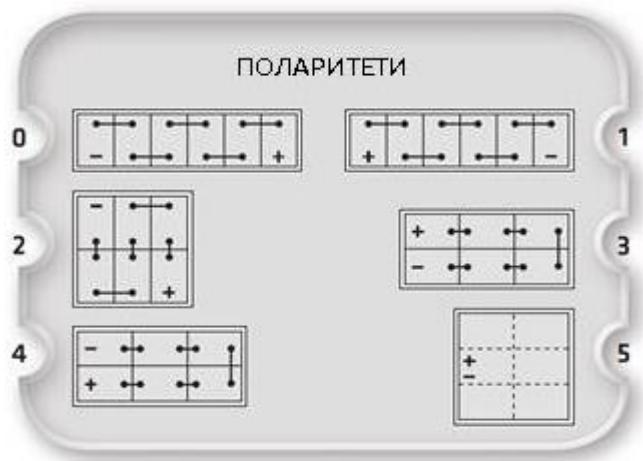
Слика број 1 : Поларитет акумулатора
