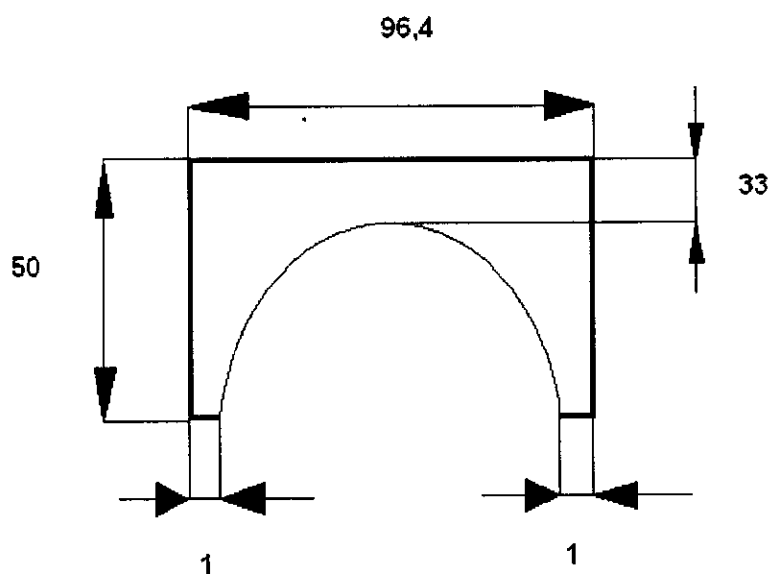
Скица 1. 96,4 x 50 (исећи полукруг, АБС на полукругу)
