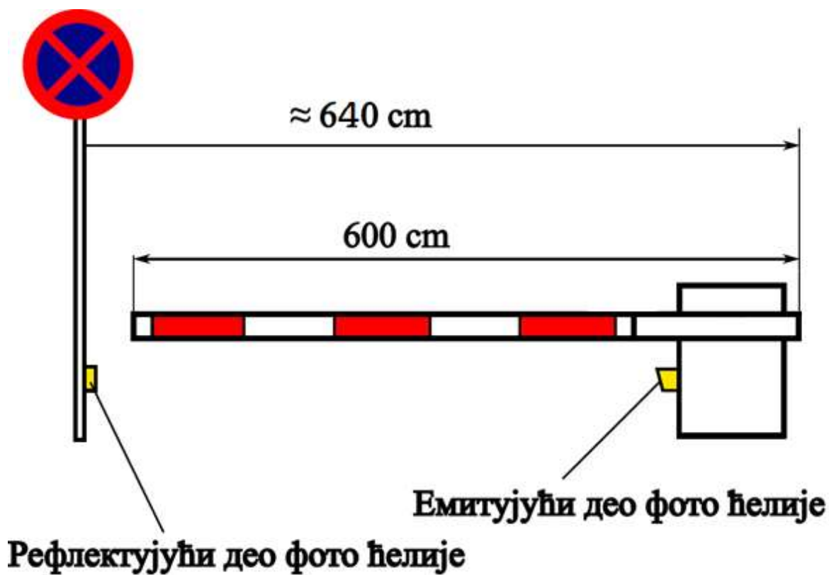
Слика 3. Скица са димензијама (стубић би стајао до саобраћајног знака или би био инсталиран на знак као носач)
