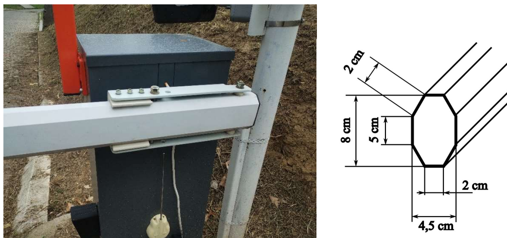
Слика 1. (а) Везивање летве са носачем и (б) попречни пресек постојеће хаварисане летве
