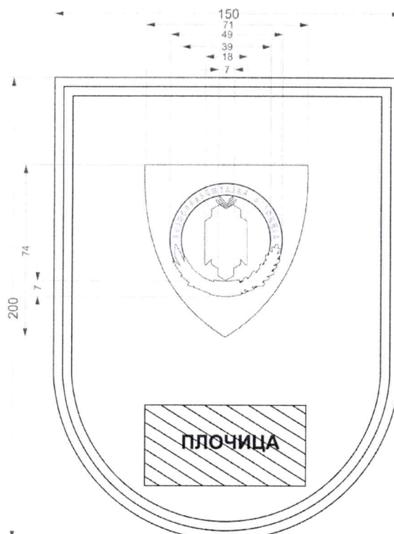
Слика 14. Димензије Плакете Војнообавештајне агенције
