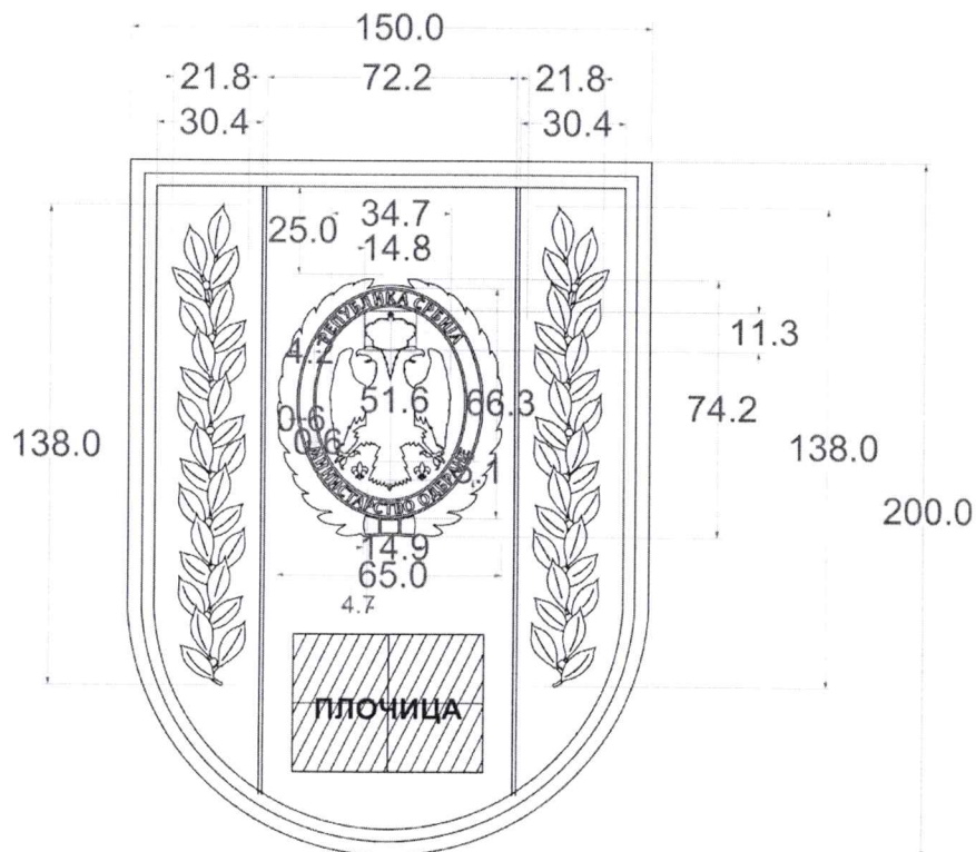
Слика 6. Димензије Плакете Министарства одбране
