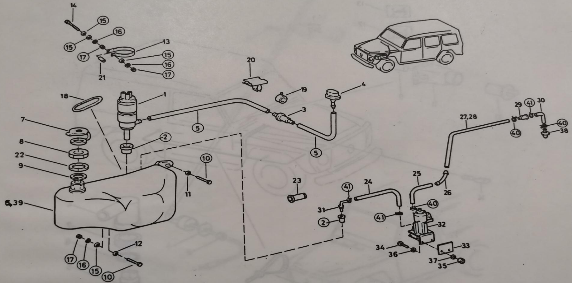
Sl. 157 — Uređaj za pranje stakla (190.10.02)
