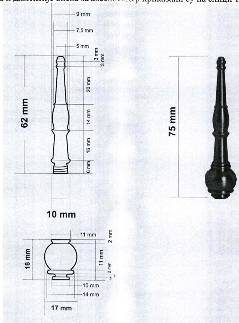
Слика 1 – Спољни изглед и димензије виска за акселбендер
